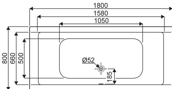
Baignoire 180x80 réf : 000893 00 000
